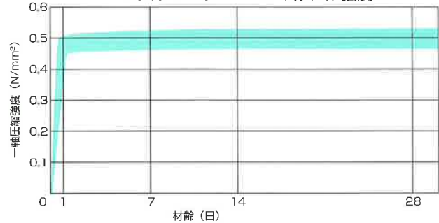
シリカジョイン M70 の砂ゲル強度
