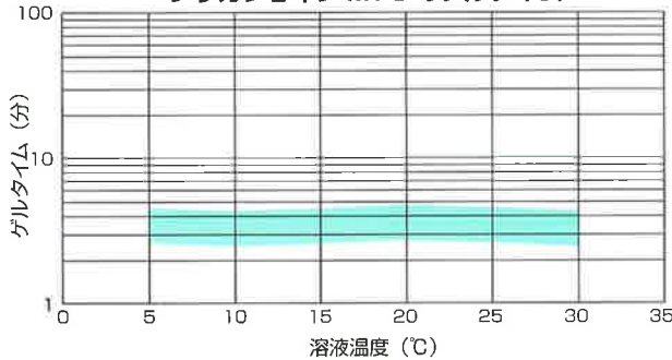
シリカジョイン M70 のゲルタイム
