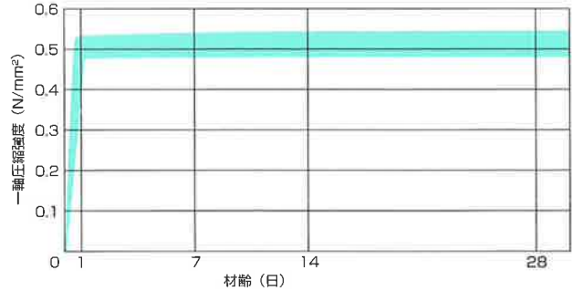
シリカジョイン S70 の砂ゲル強度
