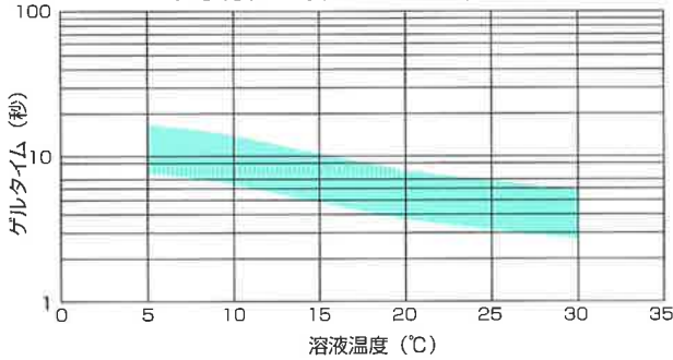
シリカジョイン S70 のゲルタイム
