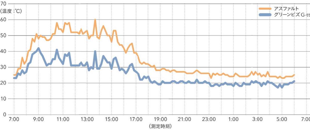
グリーンビズ G-tt とアスファルト舗装の表面温度推移グラフ。外気温が上がる日中で特に温度差が大きくなっており、グリーンビズ G-tt 舗装は約20℃の低減効果を発揮している。
