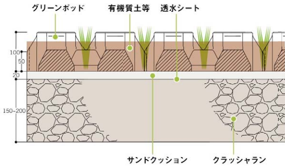
▼ 施工断面図 空隙部に芝が根を張ることができ、芝枯れを防ぎます。
